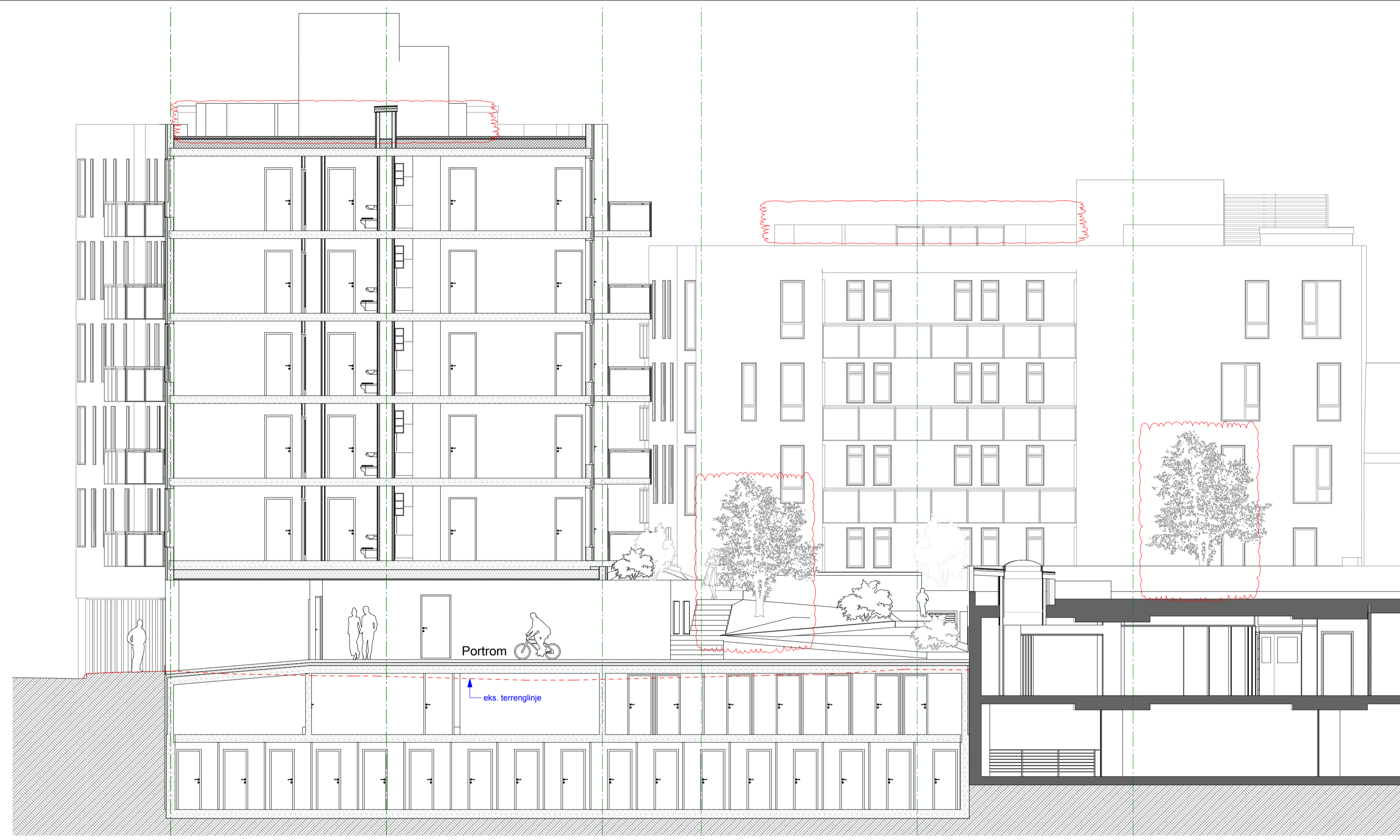
Snitt C 1:100
