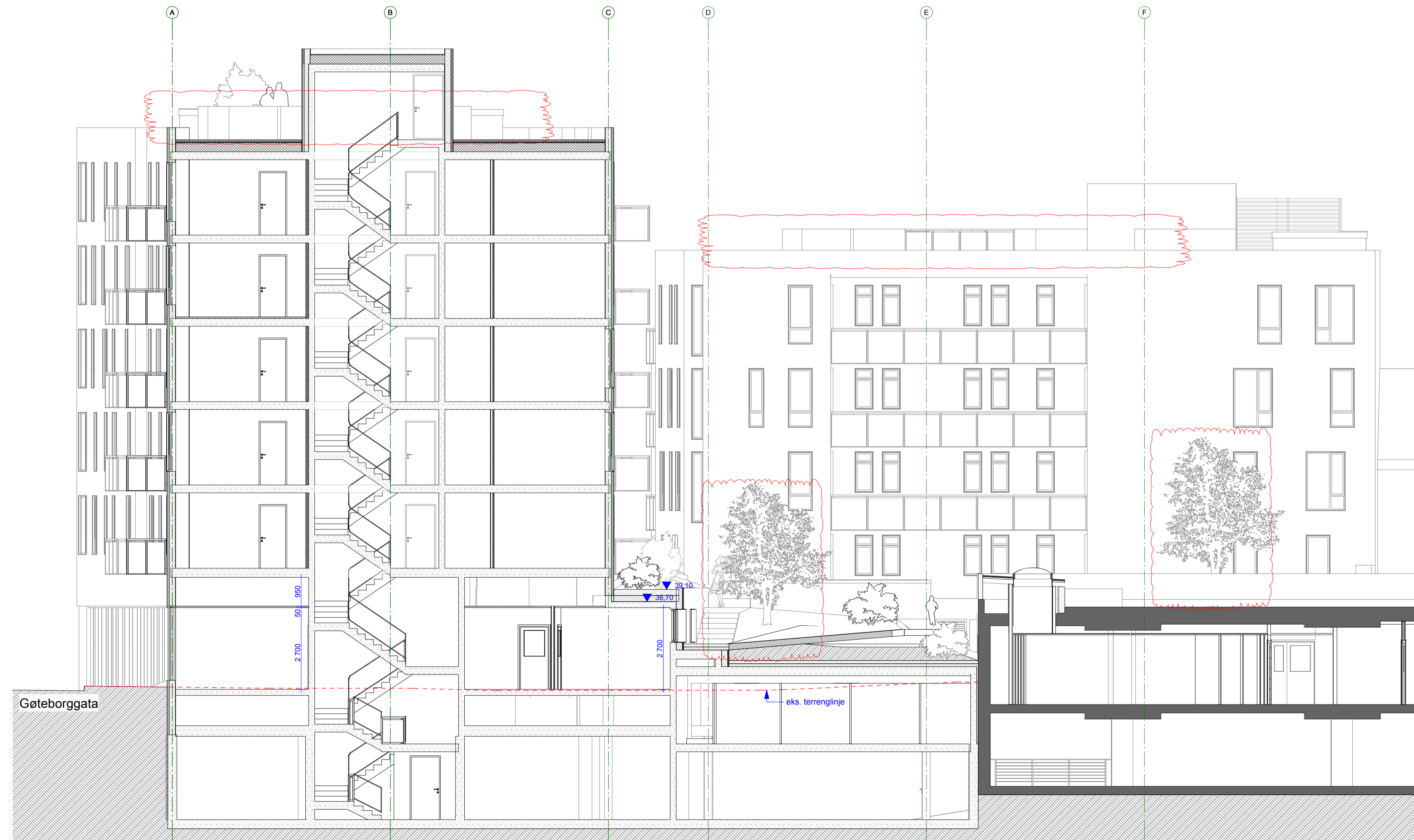
Snitt D 1:100
